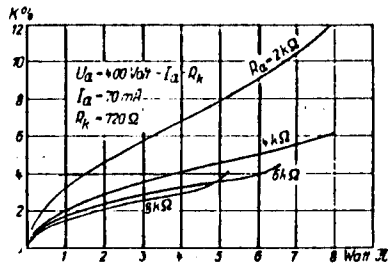
Klirrfaktor als Funktion der Nutzleistung für Eintakt-A-Betrieb. Parameter R_a
