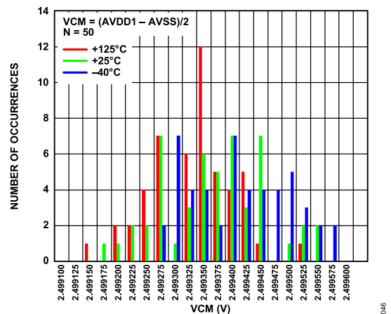
Figure 45. VCM Output Voltage Distribution, V_{CM} = (AVDD1 - AVSS)/2
