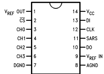
ADC08034
