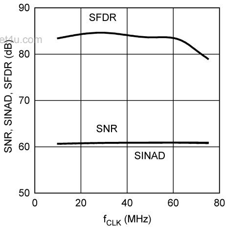
SNR, SINAD, SFDR vs. f_{CLK}
