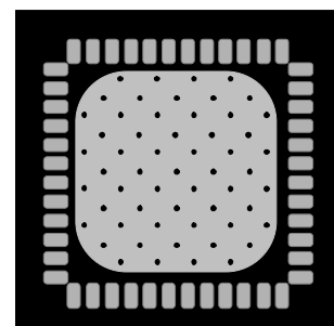
SOLDER MASK-TOP LAYER
