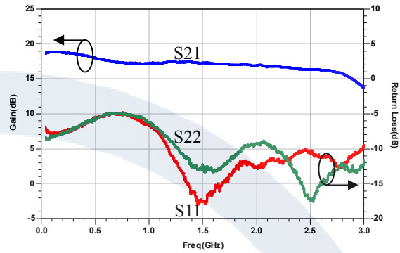
S-Parameter
