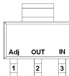
SOT-223
