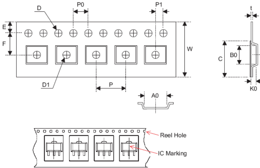
SOT89
