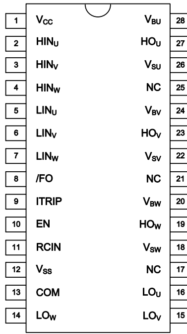
SOP-28L
