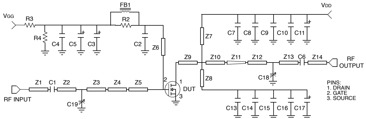
A. Schematic
