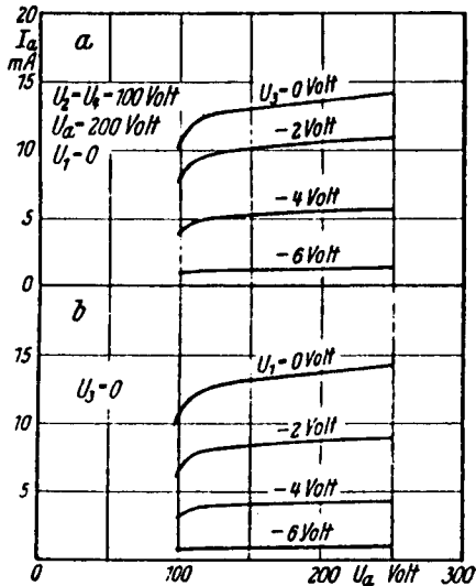
Anodenstrom-Anodenspannungs-Kennlinien
