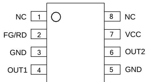
M8 Package (MSOP-8)
