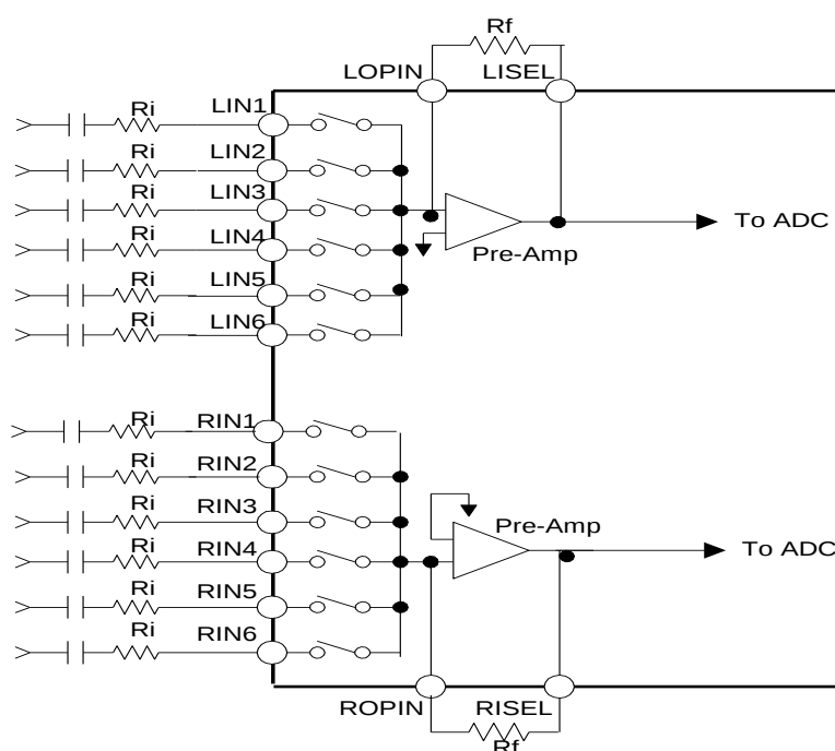
Figure 21. Input ATT
