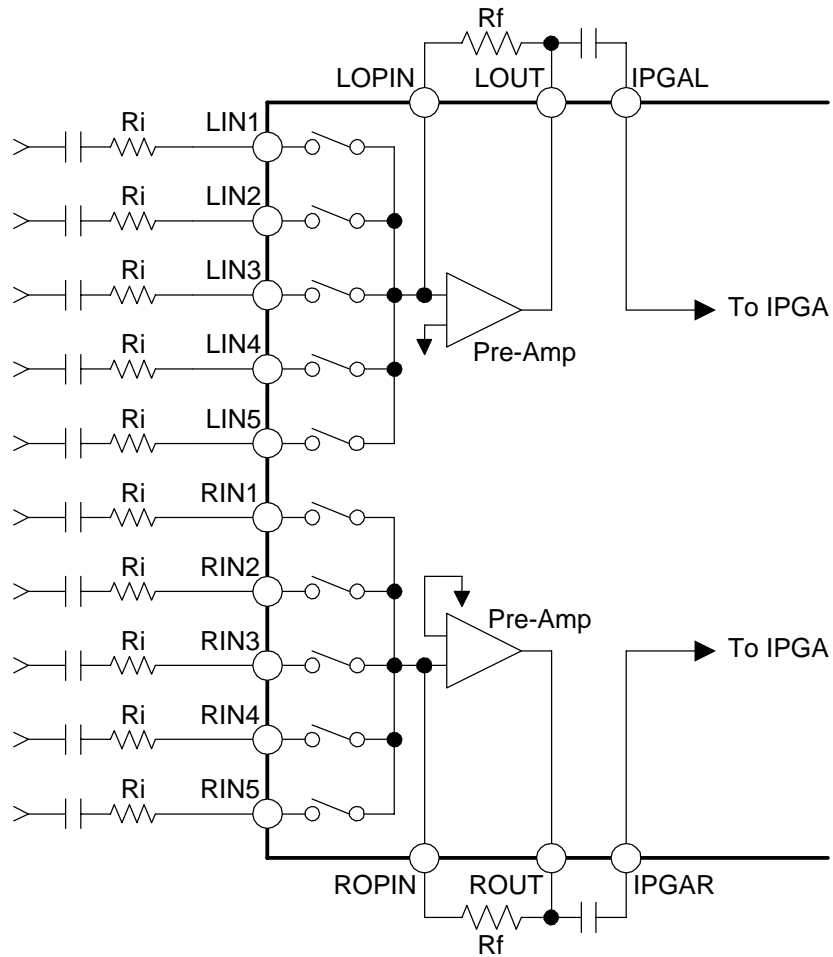
Figure 7. Input ATT
