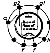
Sockelschaltschema
