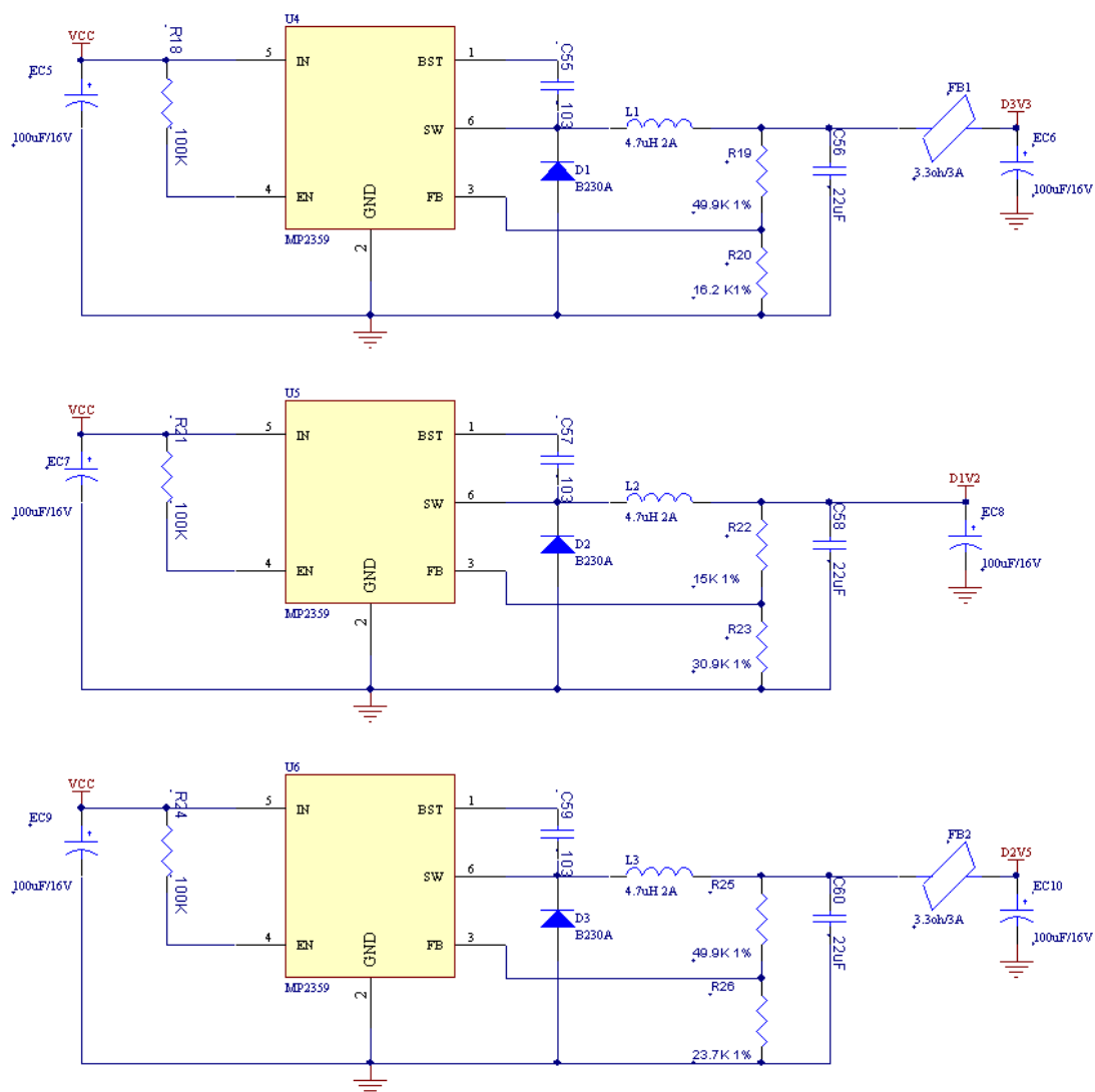
电源部分原理图
