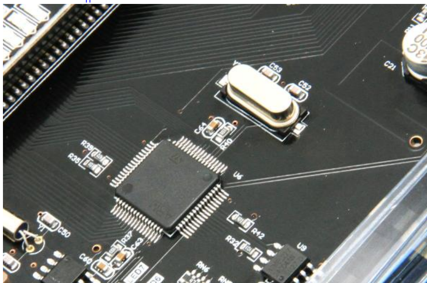
STM32F103 实物
