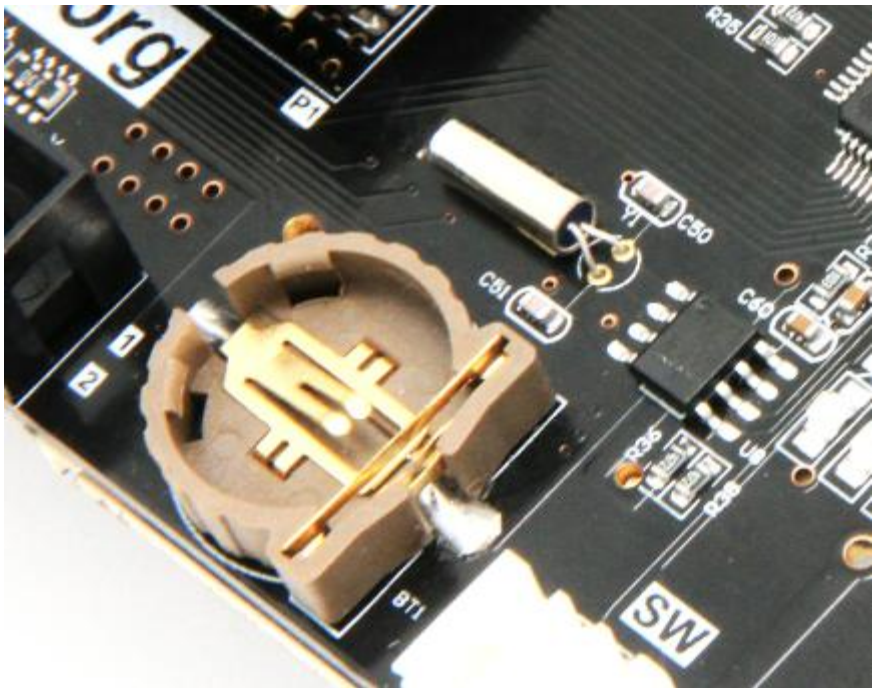
实时时钟 实物图
