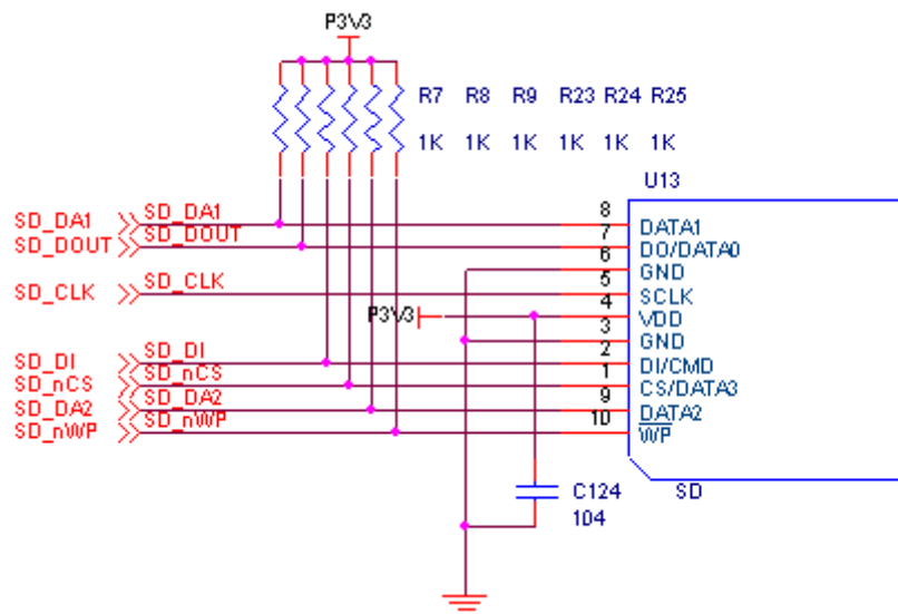
SD 卡 原理图
