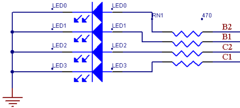
LED 原理图
