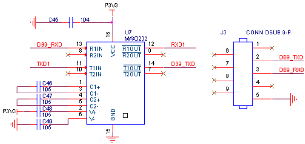
串口原理图
