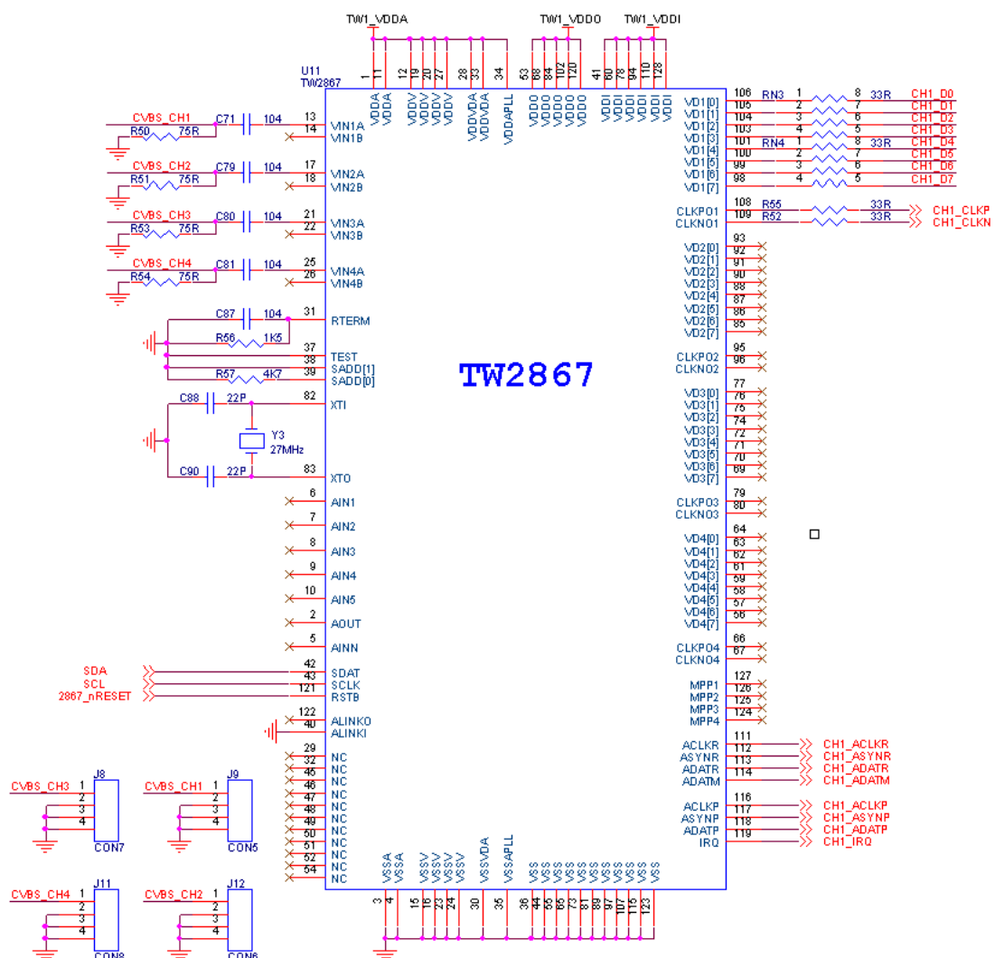
视频输入接口原理图
