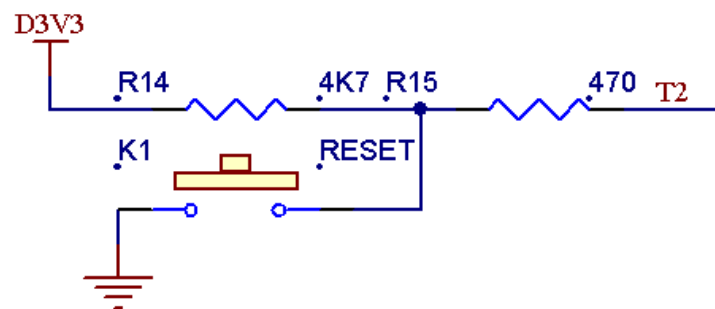
复位按键原理图
