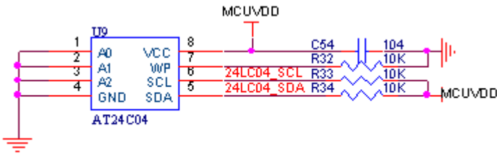
EEPROM 原理图
