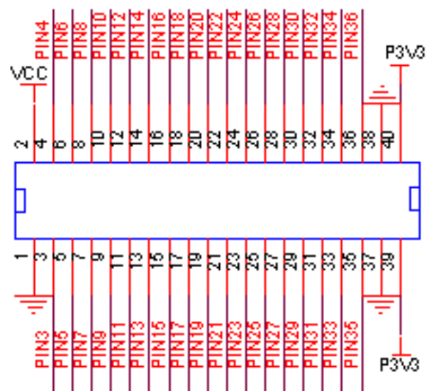
扩展口 原理图
