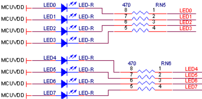
LED 原理图
