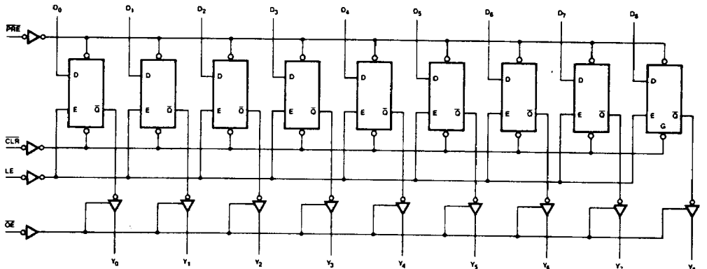
Am29843
