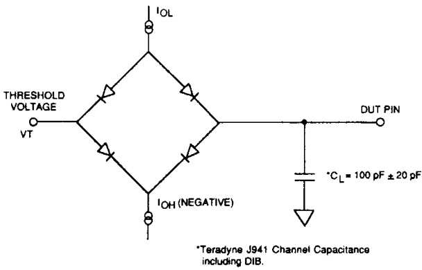
A. Standard Dynamic Load
