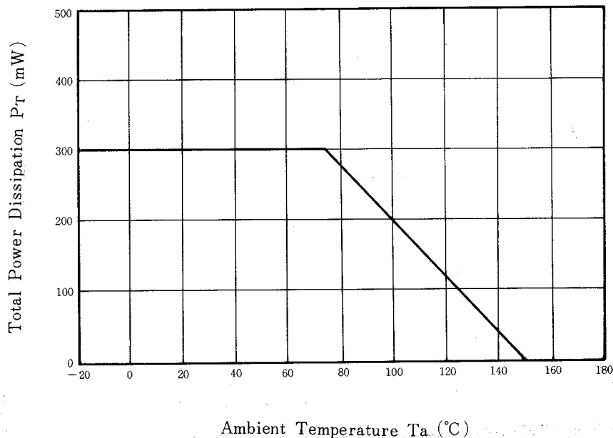
P_T - T_a
