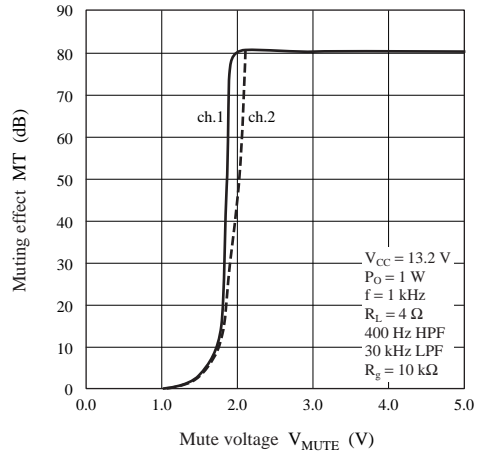
MT — V_{MUTE}
