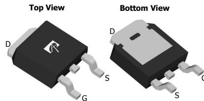
TO252 DPAK
