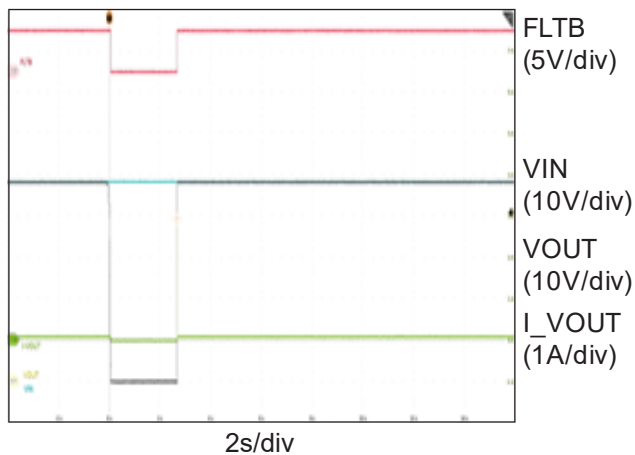
Thermal Shutdown (-01)
