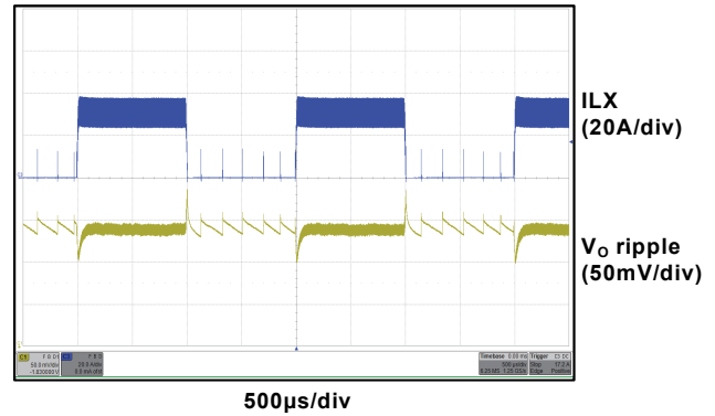
Load Transient 0A to 30A
