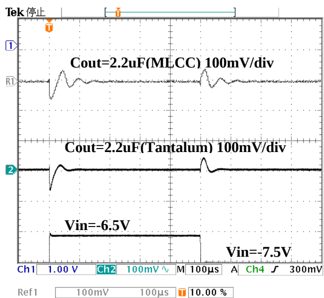
■Cin=1.0uF(Tantalum) Iout=5mA
