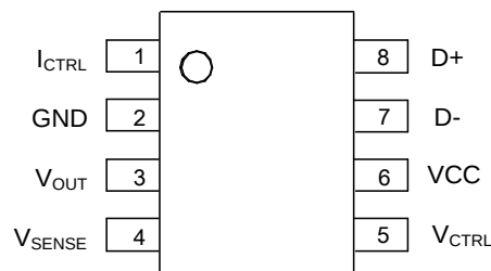
SO-8
