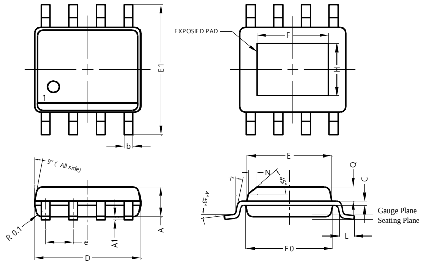
SO-8EP
