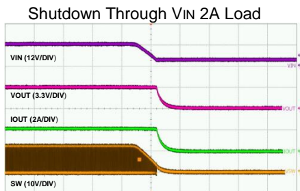
Time-200μs/div
