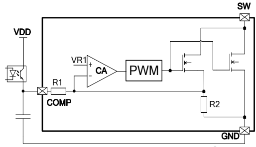
图 2. 反馈电路
