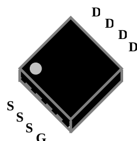
PMPAK ® 3 x 3
