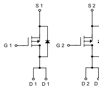
P-Channel MOSFET
