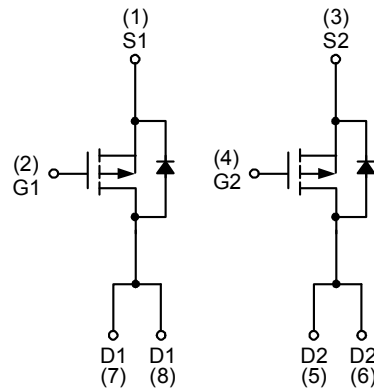
P-Channel MOSFET
