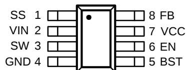
APW7512 TSOT-23-8A
