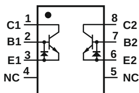
AS194DE AS394DE, AS394CDE SOIC-8 (150mil) / EPAD
