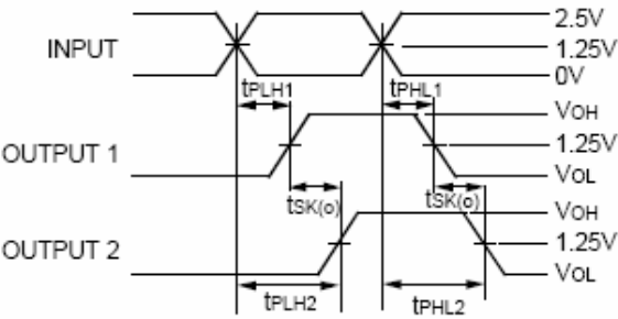
Output Skew - tSK(O)
