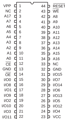
SOIC (SOP)
