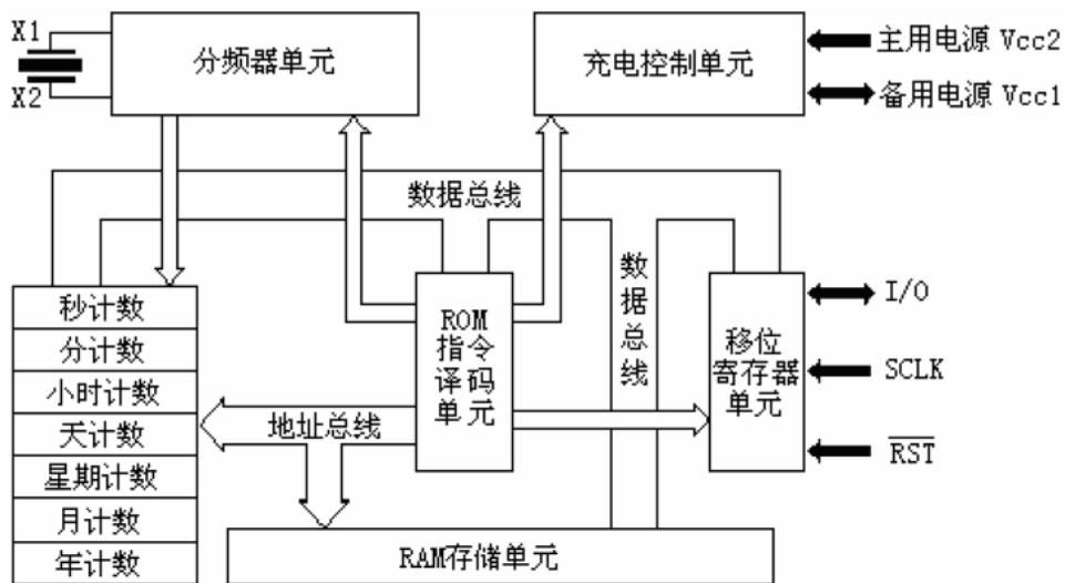
图1 AT8303内部框图
