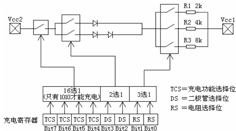
图4 AT8303 可编程慢速充电器
