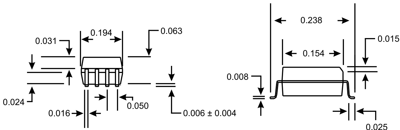
8 - Pin SOIC
