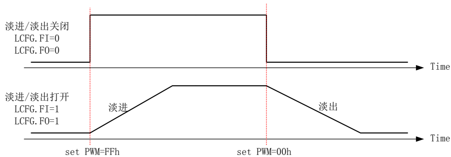
图 7 PWM 控制模式下的“淡进”和“淡出”功能
