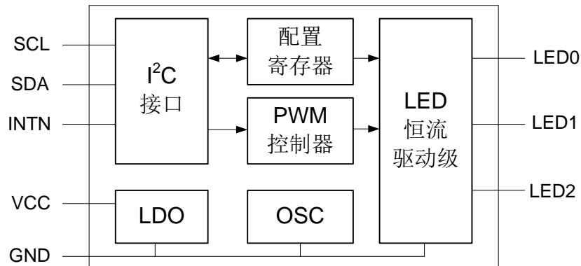
图 2 AW2013 框图
