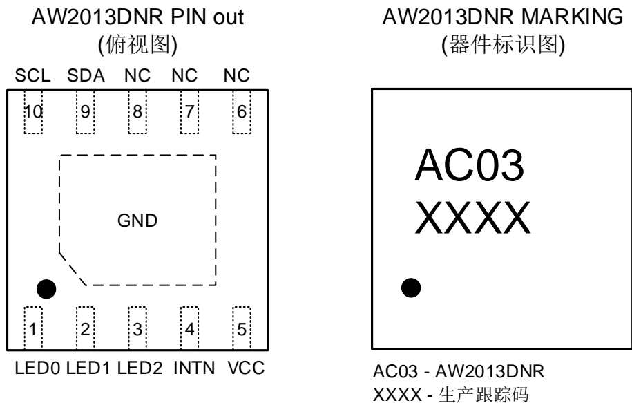
图 3 AW2013 引脚分布及标记图 (俯视图)
