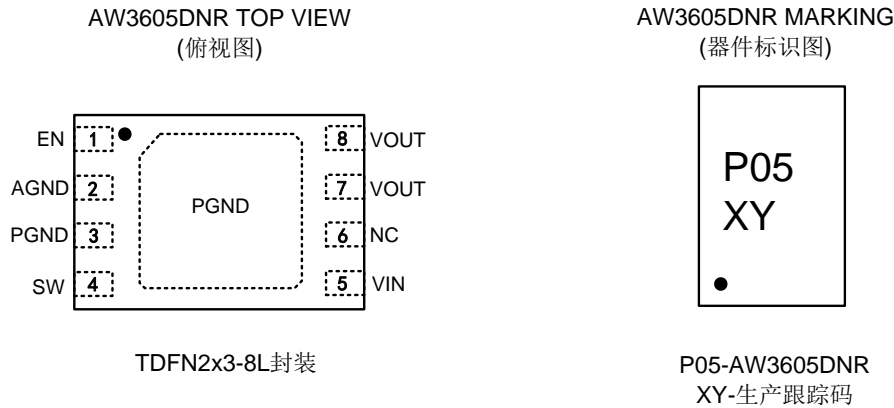
图1 AW3605DNR 引脚分布俯视图及器件标识图
