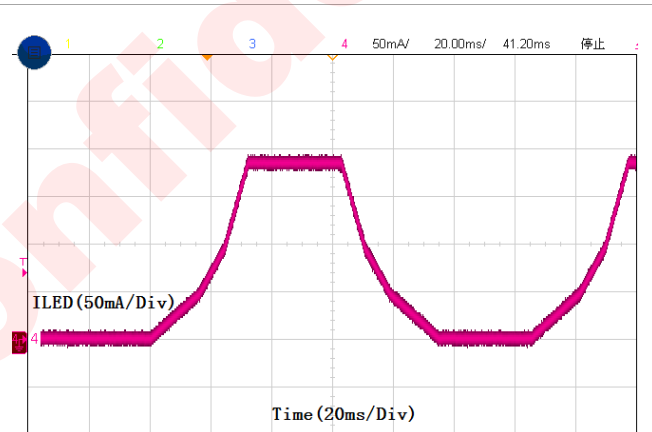
ILED=187.5mA log mode
