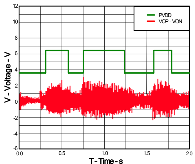
图 4 AW8733 chargepump 输出随输入变化波形
