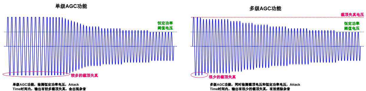
图 9 单级 AGC/多级 AGC 工作原理图
