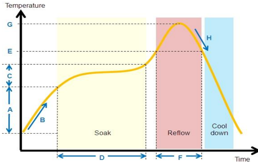
图 10-1 AXP313A 典型回流焊曲线
