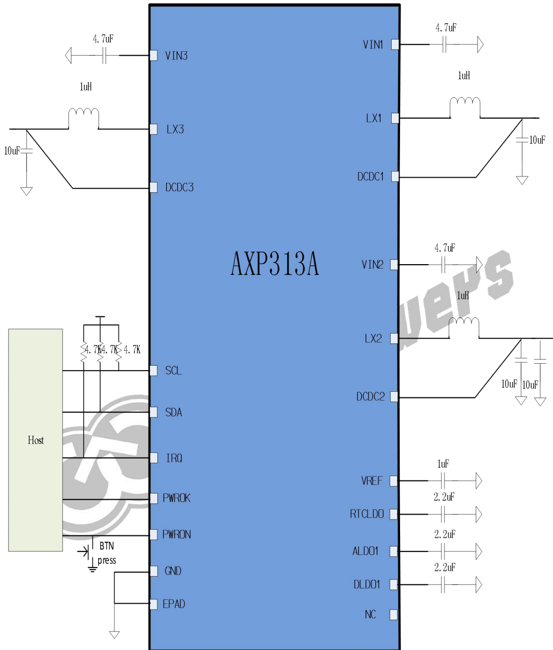
图 7-1 典型应用图
