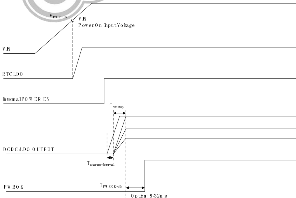
图 6-2 开机时序
