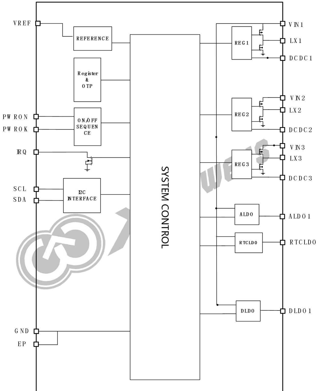
图 6-1 结构框图
