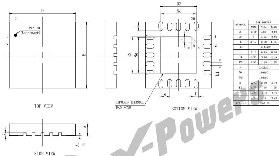
图 9-1 封装信息
