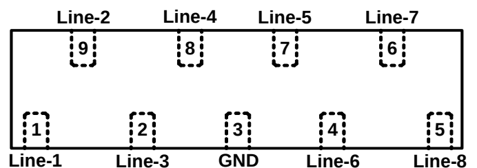
DFN3810P9E (Top View)
