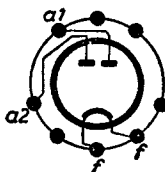
Sockelschaltenschema
