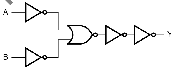
图 3 逻辑框图
