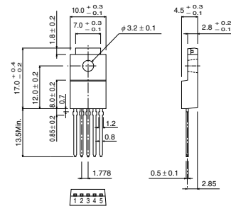
TO220FP-5
