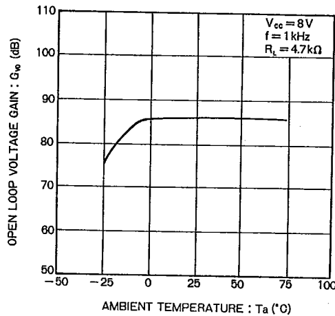
Fig. 12 開回路電圧利得—周囲温度特性
