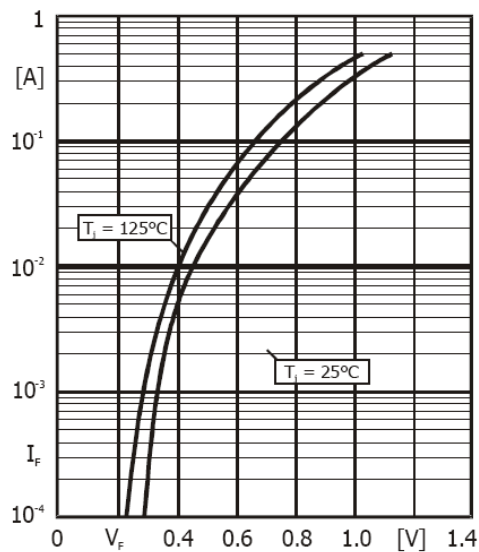
Forward characteristics (typical values) Durchlasskennlinien (typische Werte)
