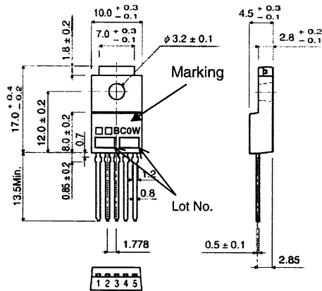
TO220FP-5 (UNIT : mm)
